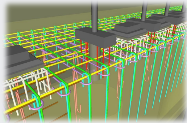
橋台支承部干渉チェックモデル
