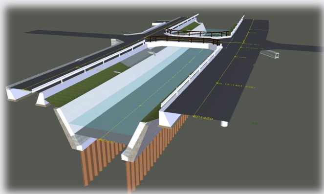
橋梁・河川護岸統合モデル
