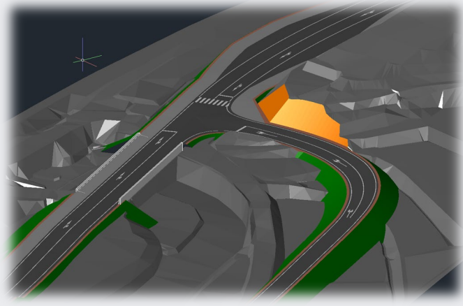
交差点設計 (道路線形モデル)
