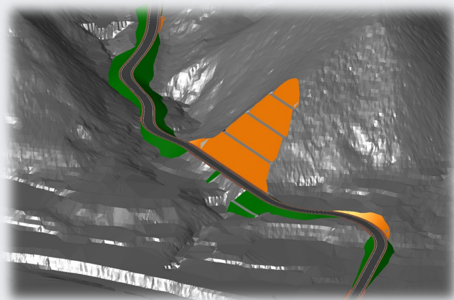
工事用道路 (道路線形モデル)
