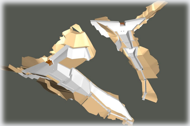
砂防堰堤・土工形状統合モデル
